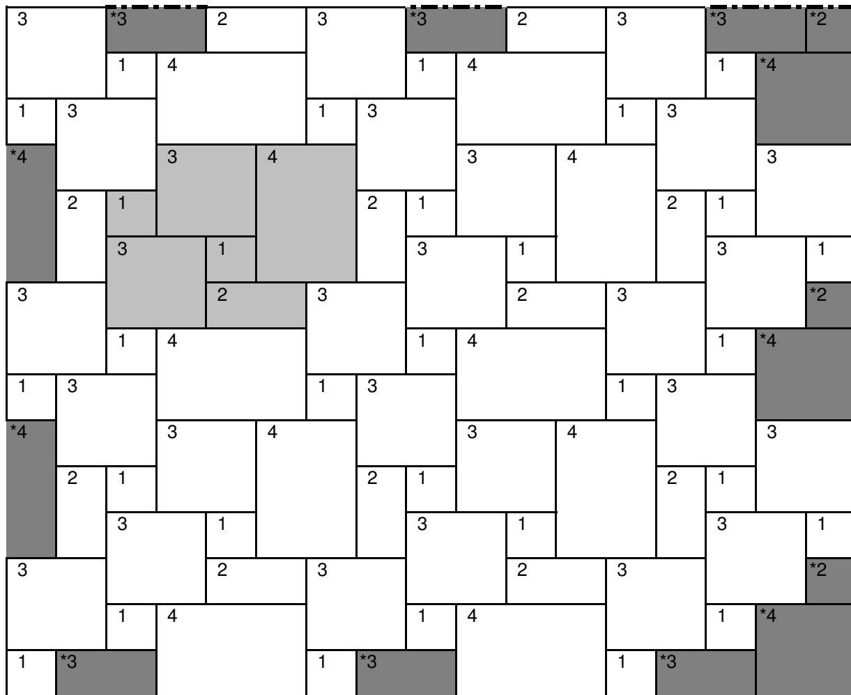
Groot Romaansverband met als grootste tegel 60*90
